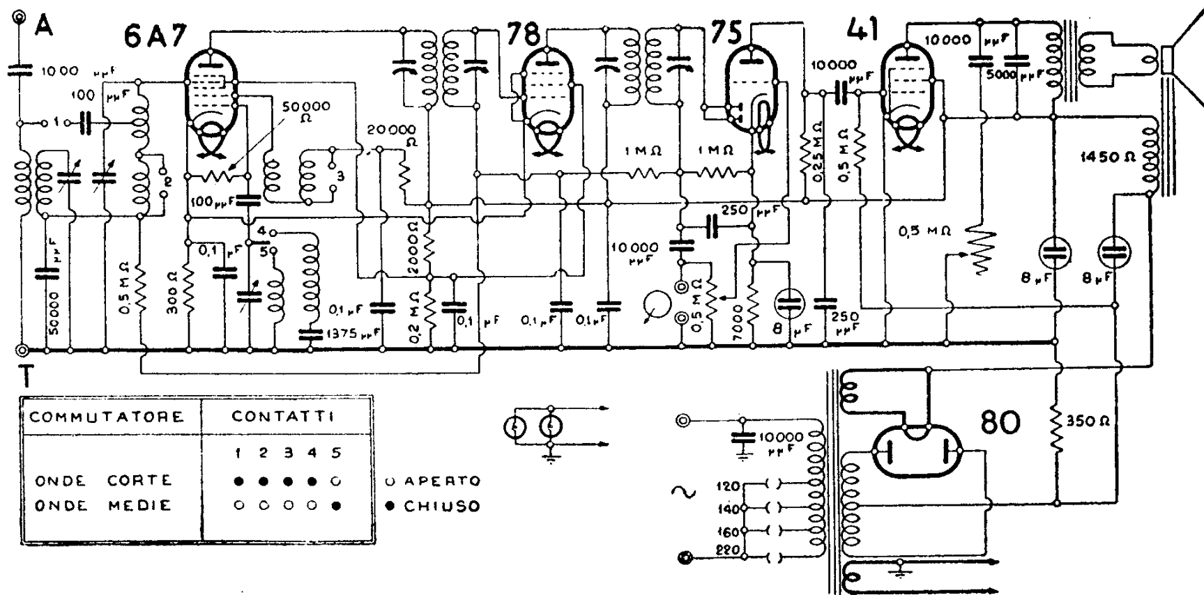
WATT RADIO - MOD. « ONDINA V »
